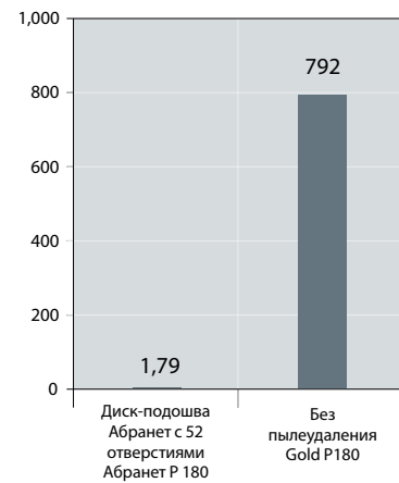
Количество пыли на окружающих поверхностях (г/кг)
